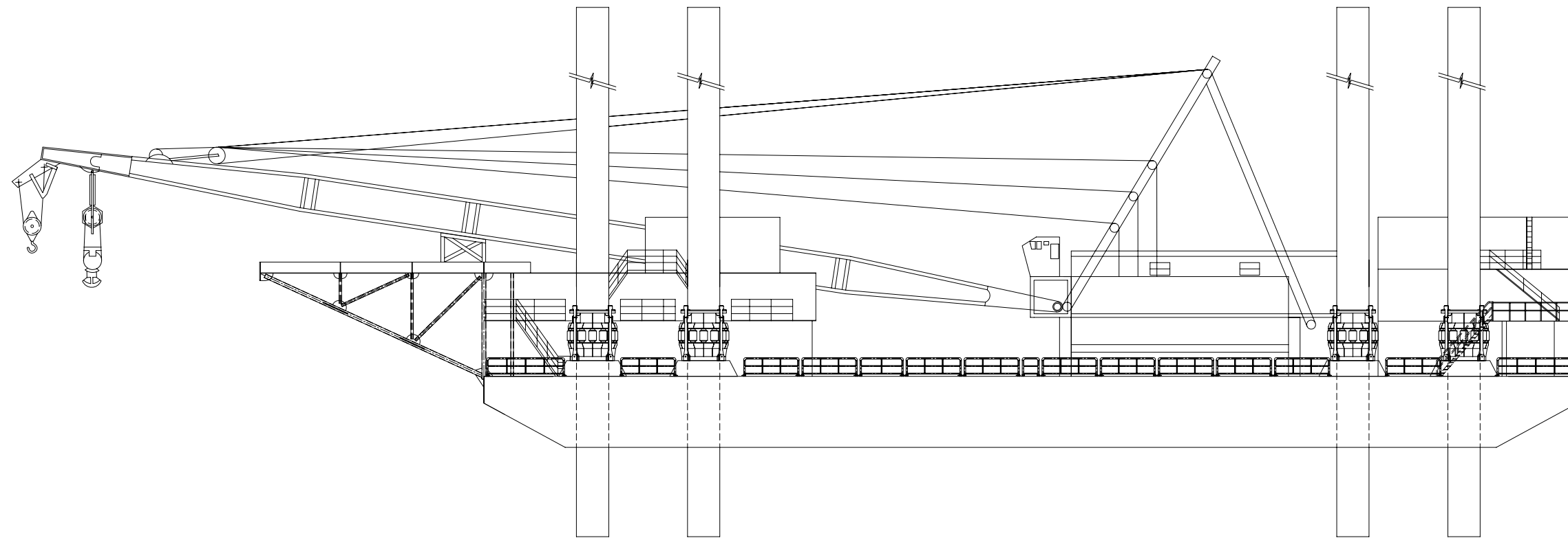
ELEVATION
